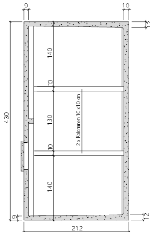
COUPE LONGITUDINALE
