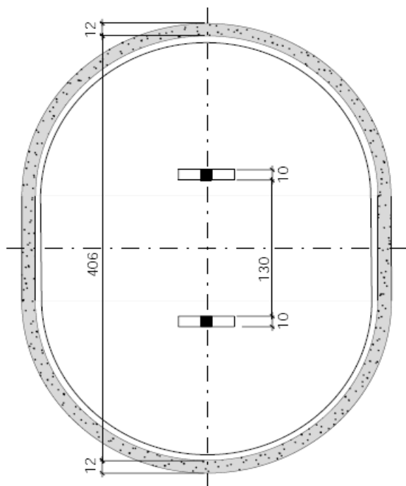
SEMELLE : COUPE HORIZONTALE
