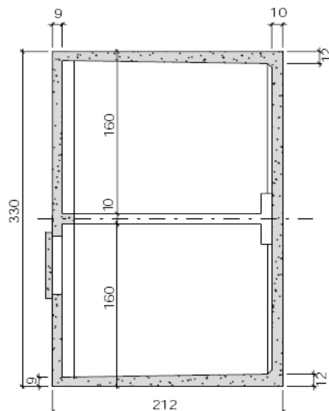
COUPE TRANSVERSALE
